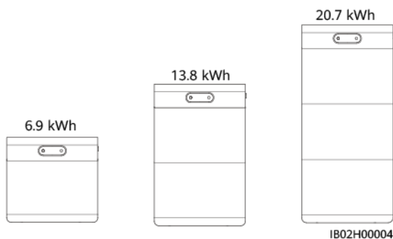
Afbeelding2-4 Capaciteitsuitbreiding met Energy Storage Modules
