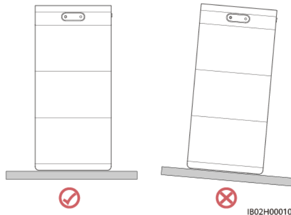
Afbeelding4-2 Installatiehoek
