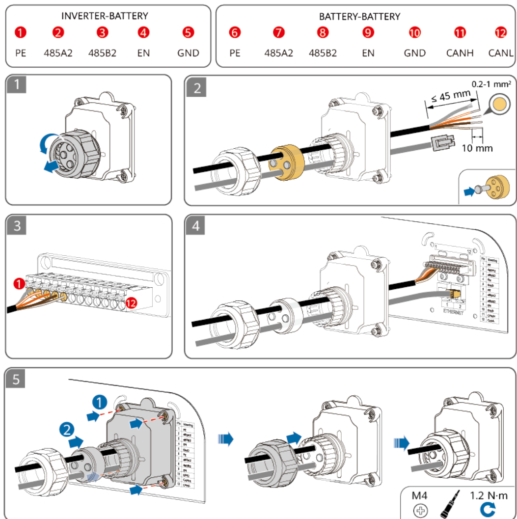
Afbeelding5-7 Signaalpoortansluitingen
