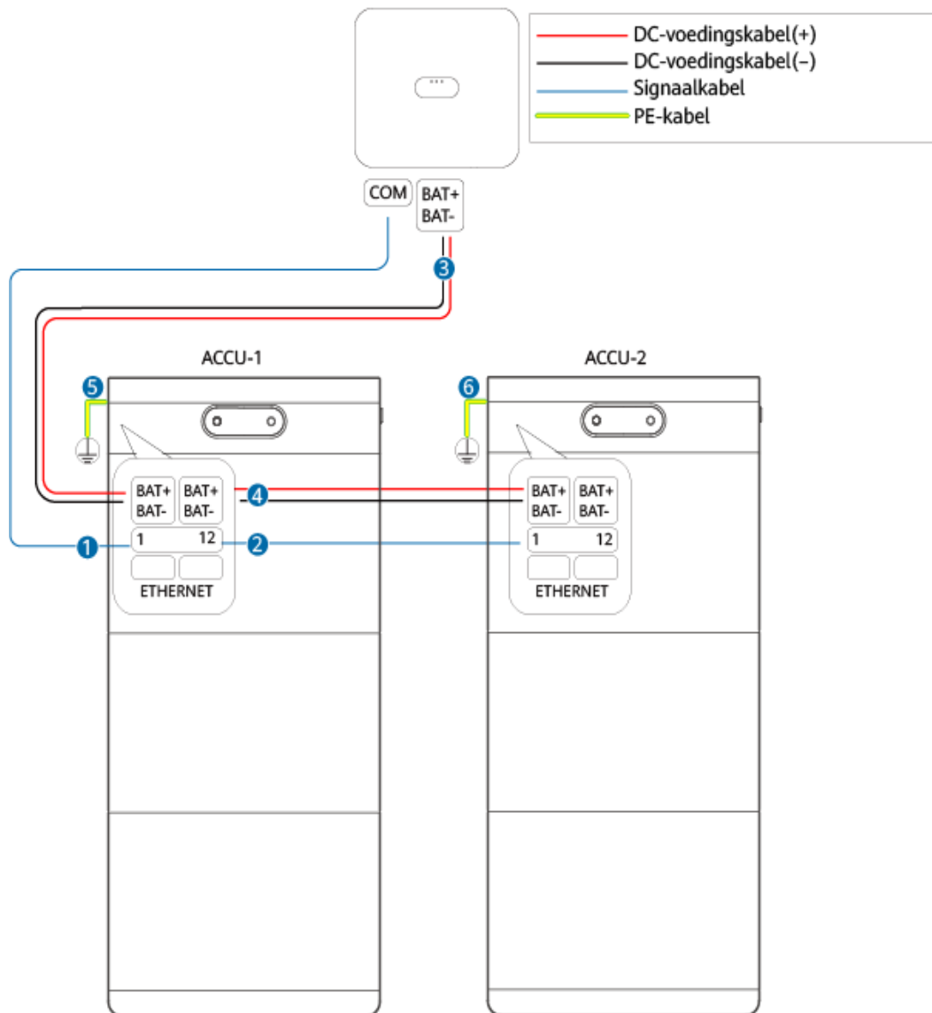
Afbeelding5-1 ESS-kabelaansluitingen
